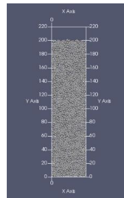
図-2. 空中落下法による粒子充填
