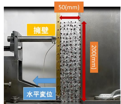
図-1. 変形前の擁壁とアルミ棒積層体
